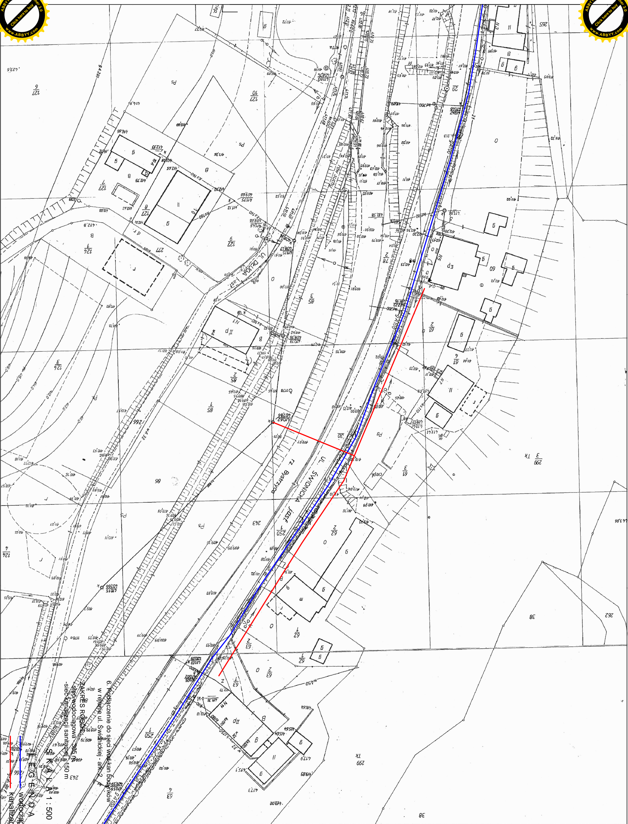
KOPIA MAPY ZASADNICZEJ SKALA 1:500
